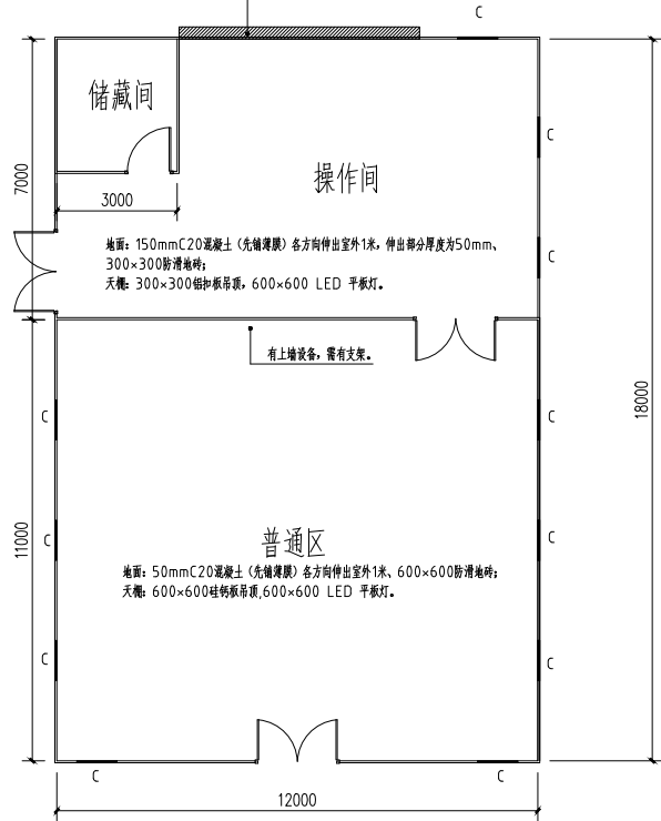
平面图
